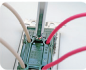
連結端子に。
